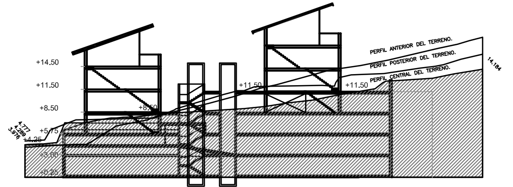
-PROPOSTA ESQUEMATICA DE SECCION TRANSVERSAL-
