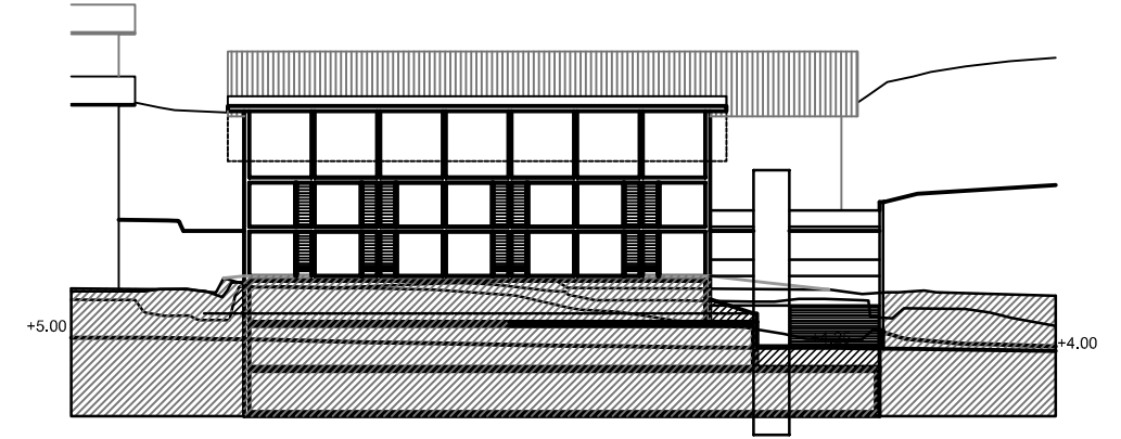
- ESQUEMAS SECCIONES TRANSVERSAL Y LONGITUDINAL -
