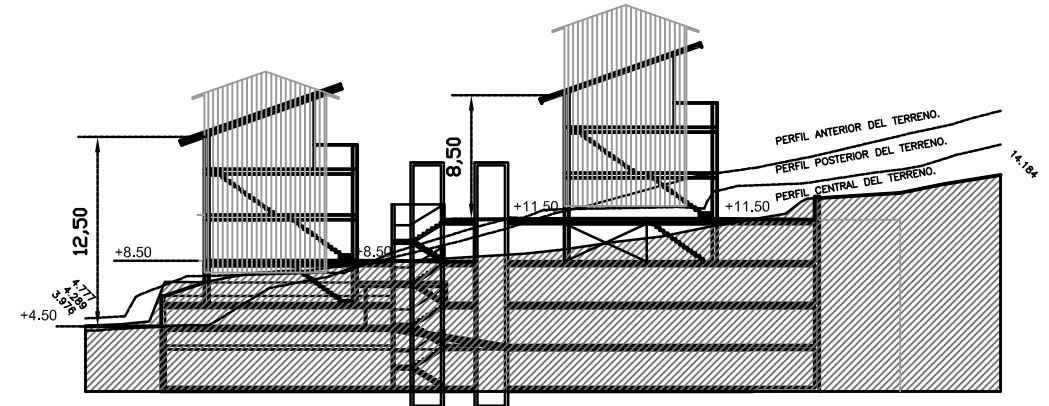
- ESQUEMAS SECCIONES TRANSVERSAL Y LONGITUDINAL -
