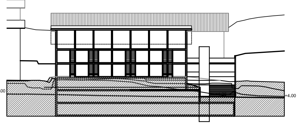
- ESQUEMAS SECCIONES TRANSVERSAL Y LONGITUDINAL -
