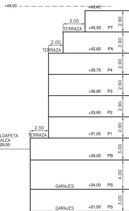
PERFIL NORMATIVO 6 PLANTA BAJA+4 PLANTAS ALTAS+ATICO+TORREON
