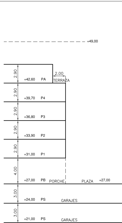
PERFIL NORMATIVO 3 PLANTA BAJA+4 PLANTAS ALTAS+ATICO
