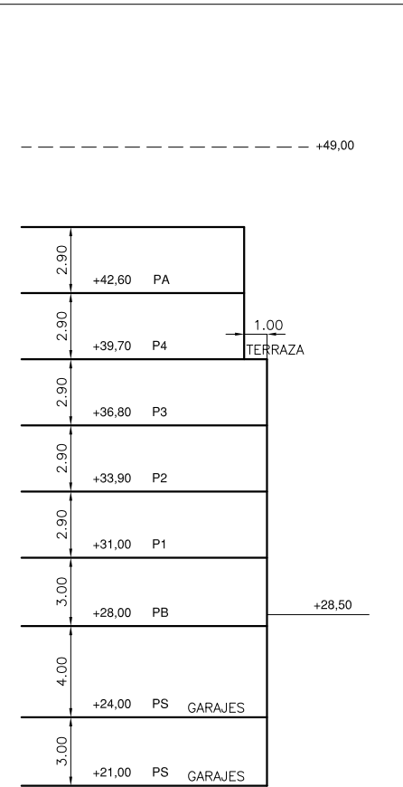
PERFIL NORMATIVO 4 PLANTA BAJA+4 PLANTAS ALTAS+ATICO
