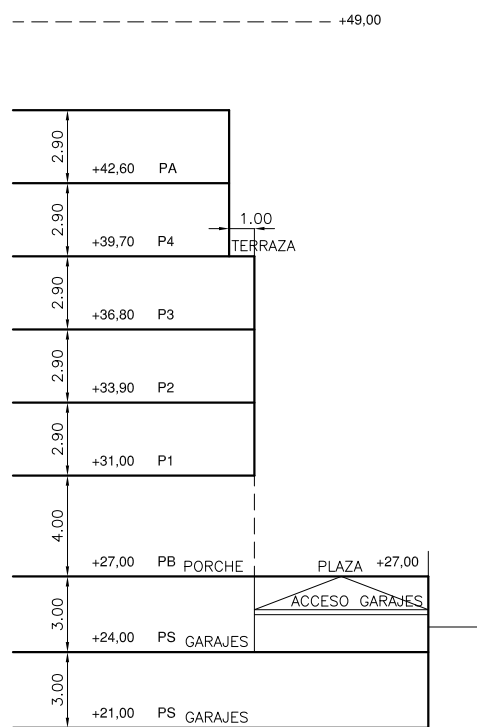
PERFIL NORMATIVO 5 PLANTA BAJA+4 PLANTAS ALTAS+ATICO
