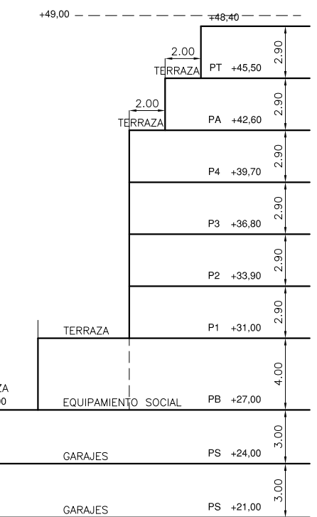
PERFIL NORMATIVO 8 PLANTA BAJA+4 PLANTAS ALTAS+ATICO+TORREON
