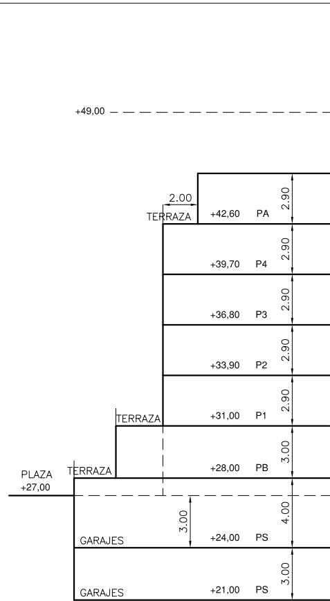
PERFIL NORMATIVO 1 PLANTA BAJA+4 PLANTAS ALTAS+ATICO
