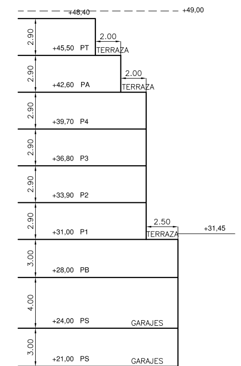
PERFIL NORMATIVO 7 PLANTA BAJA+4 PLANTAS ALTAS+ATICO+TORREON
