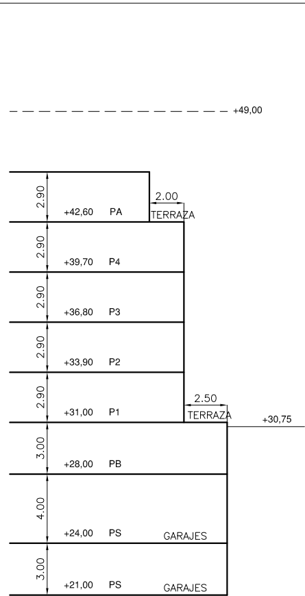
PERFIL NORMATIVO 2 PLANTA BAJA+4 PLANTAS ALTAS+ATICO
