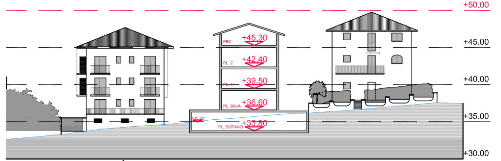
SECCIÓN CALLE LAPICE
