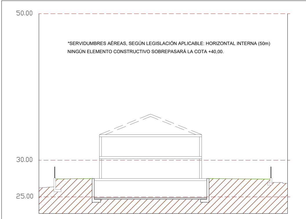
SECCIÓN. E: 1/300
