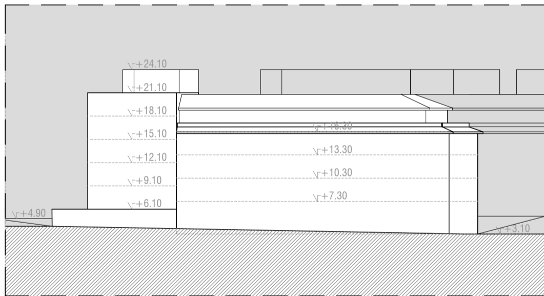
ALZADO CALLE PELEGRIN DE URANZU
