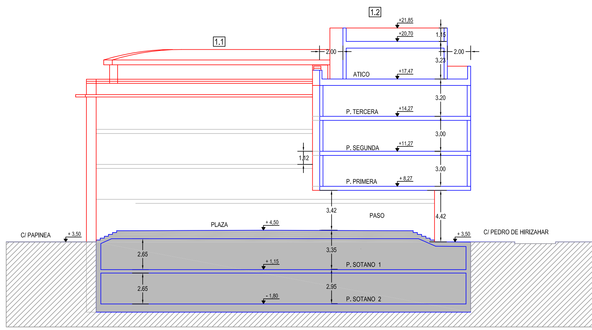
P.B.+3+AT. SECCION - S1
