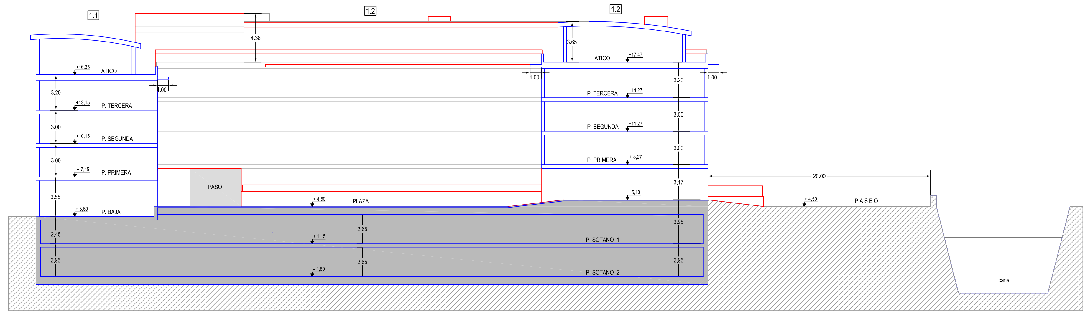
P.B.+3+AT. SECCION - S2
