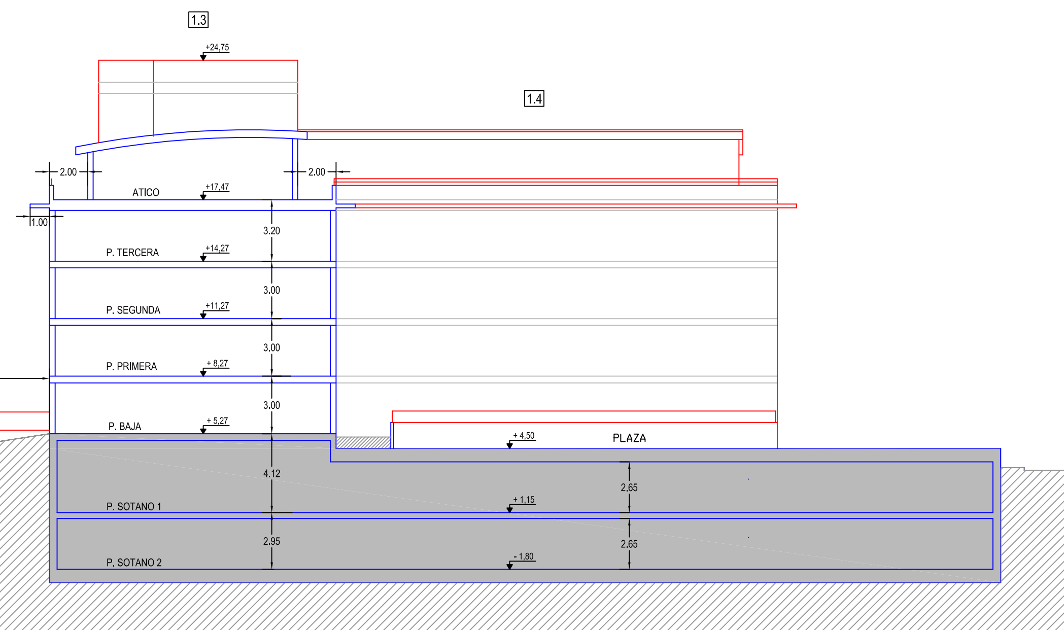
SECCION - S4
