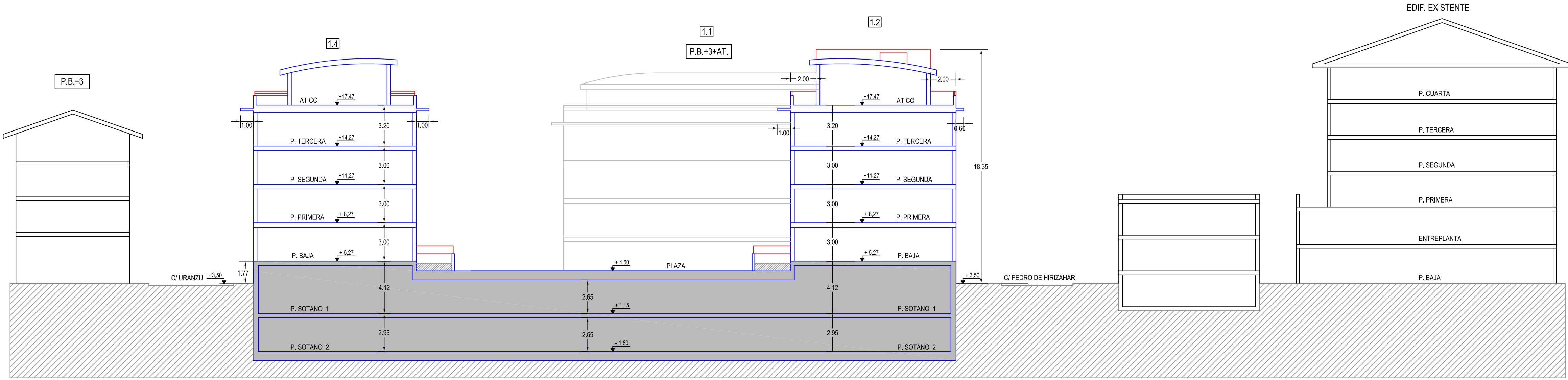
SECCION - S3
