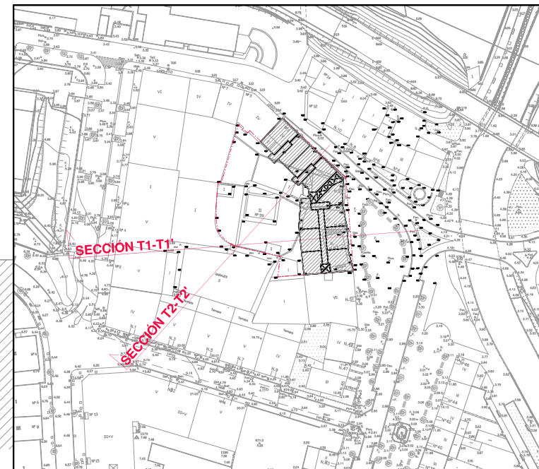
SECCION T2-T2'
