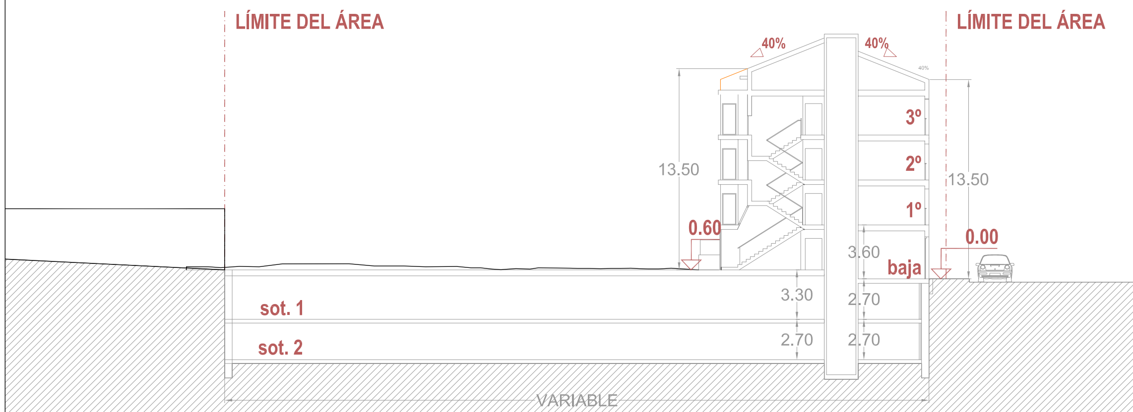
SECCION T2-T2'
