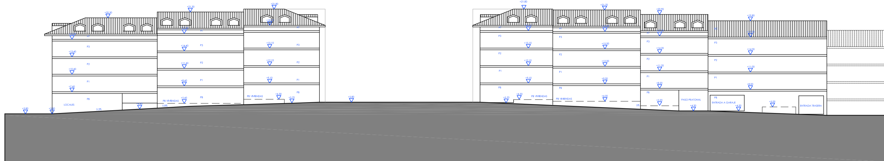
A5 - ALZADO A CALLE KORROKOITZ
