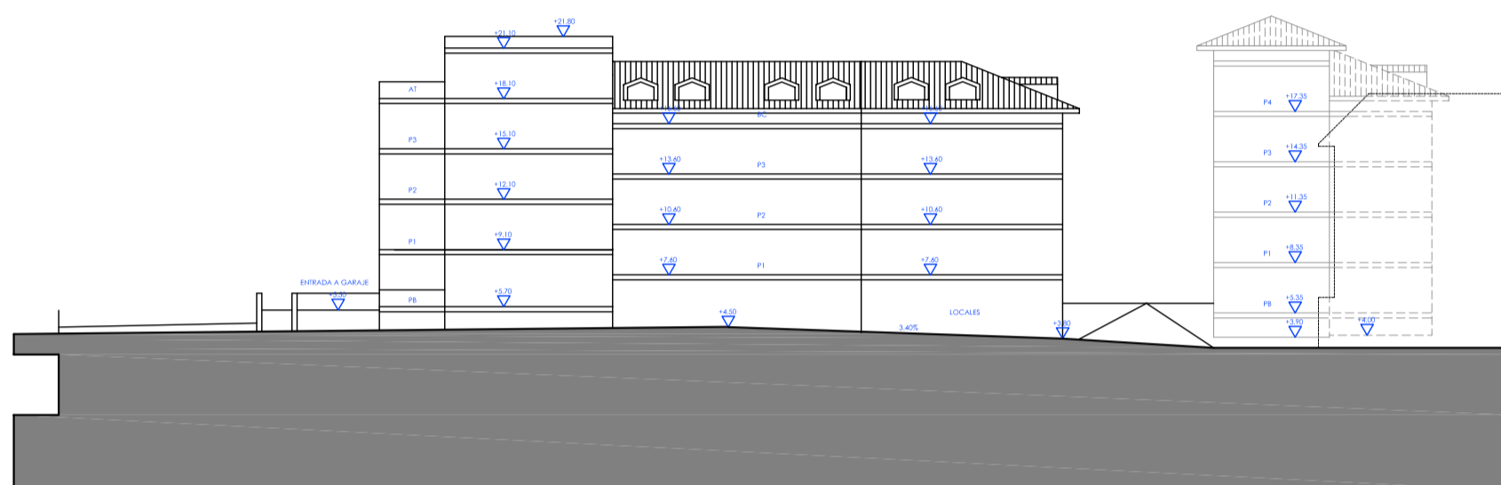
A6 - ALZADO A CALLE URANZU
