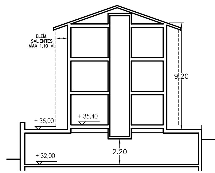
SECCION LONGITUDINAL PROYECTADA
