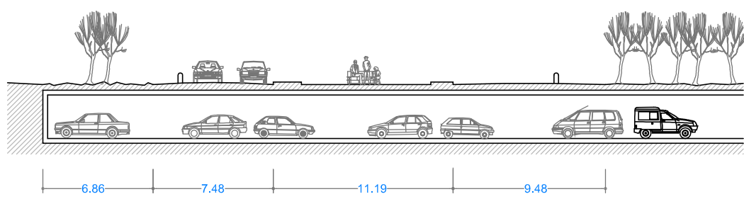
PLAZA URDANIBIA URDANIBIA ENPARANTZA E:1/300
