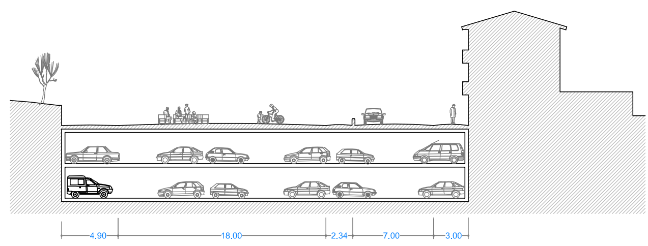
C/ JUNCAL Y PLAZA JUNKAL KALEA ETA ENPARANTZA E:1/300
