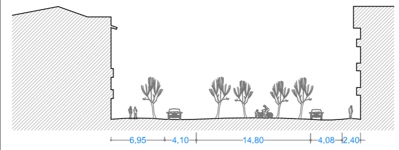
C/ SANTIAGO Y PLAZA DEL PLANTANO SANTIAGO KALEA ETA PLANTANOEN ENPARANTZA E:1/500
