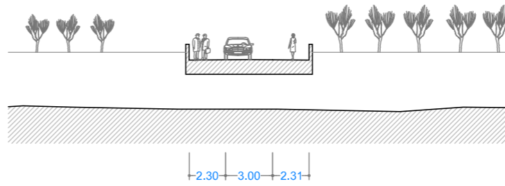
PUENTE EN LA C/ SANTA ELENA ERMITA KALEKO ZUBIA E:1/300
