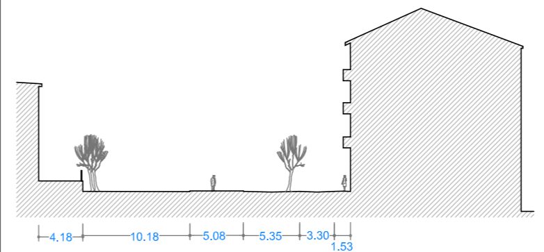
C/ ESCOLETAS ESKOLETA KALEA E:1/500
