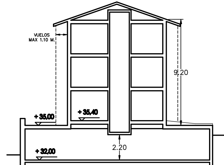
SECCION LONGITUDINAL PROYECTADA
